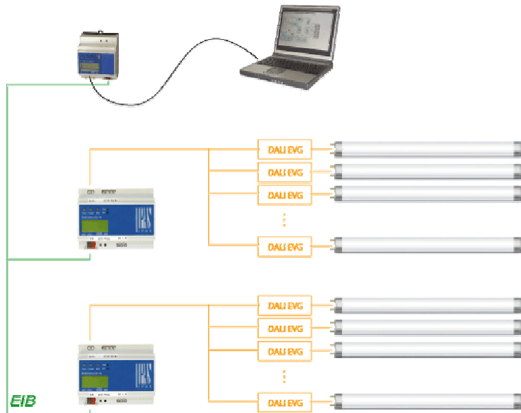
Abbildung 2 – Kommunikation über angeschlossene Schnittstelle
